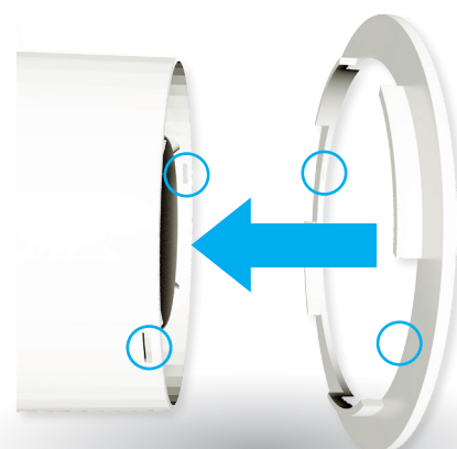
Způsob montáže na ventilátor (aretační čepy)
